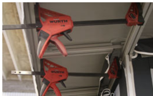
*8 - Spänn upp taket på utsidan vid frontväggen med hjälp av två tvingar.
