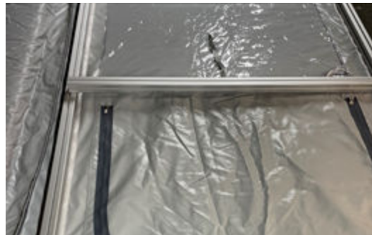
*5 - Nu är dags att trä i tvärstag nr 5, två stycken på vardera sida på bakväggen.
